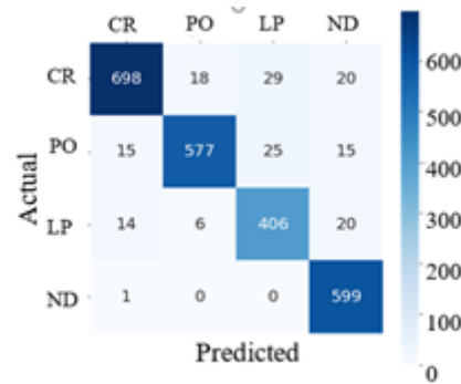
Fig. 5. Confusion matrix.
